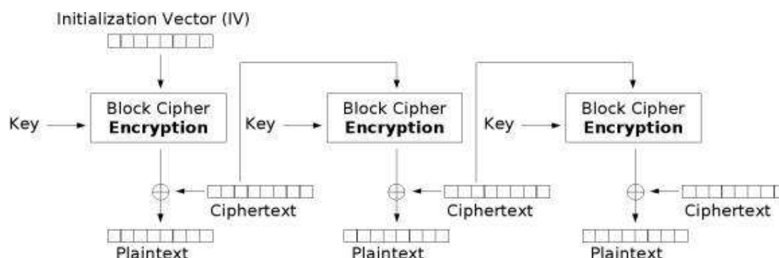
Fig. 26 Modo de des encriptación OFB (PAAR,1998)
