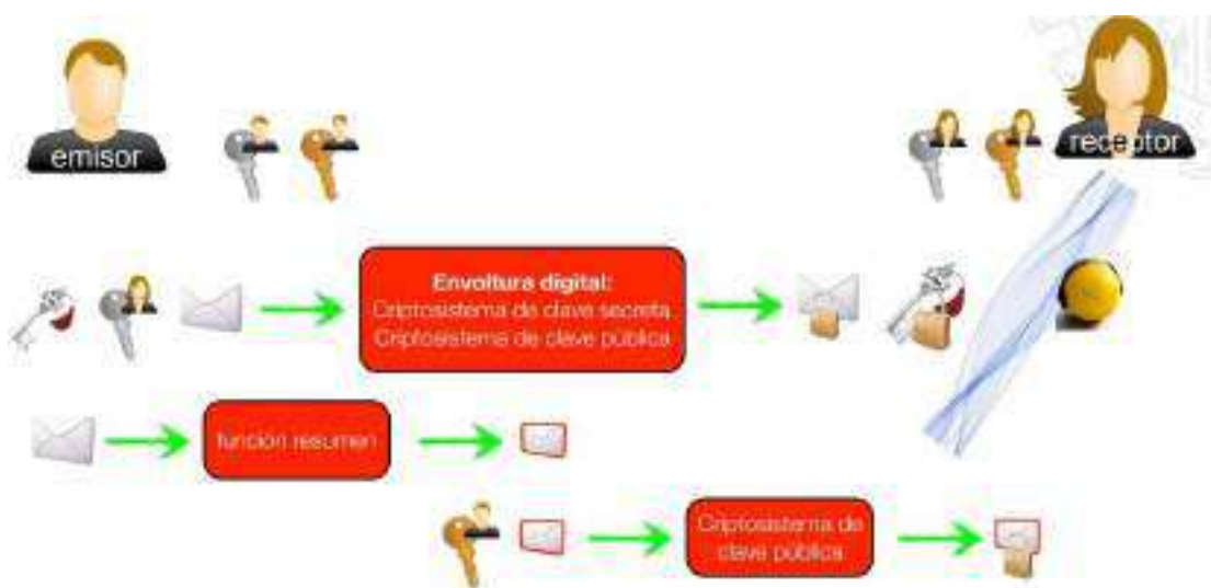
Fig. 34 Esquema de firma digital
