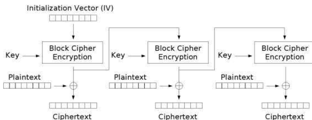
Fig. 25 Modo de encriptación OFB(PAAR,1998)
