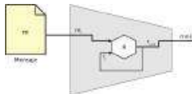
Fig27. Estructura iterativa de una función resumen. R representa la función de compresión, m es el mensaje completo, m_i el i -ésimo trozo de m , y h_i la salida de la función en el paso i (Lucena, 2010)
