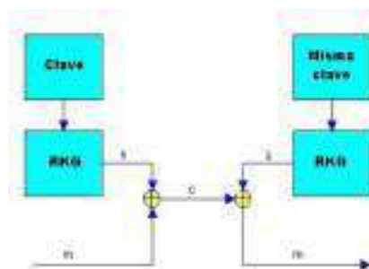
Fig. 10 Algoritmo de cifrado de flujo
