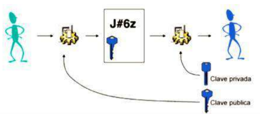
Fig. 19 Esquema de los algoritmos de clave pública
